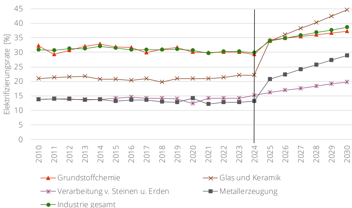
Abbildung 27: Historische und prognostizierte Entwicklung des Elektrifizierungsgrads einzelner Branchen
