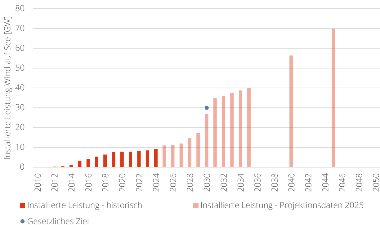
Abbildung A 14: Historische und projizierte Entwicklung der installierten Leistung von Wind auf See und die gesetzliche Zielsetzung
