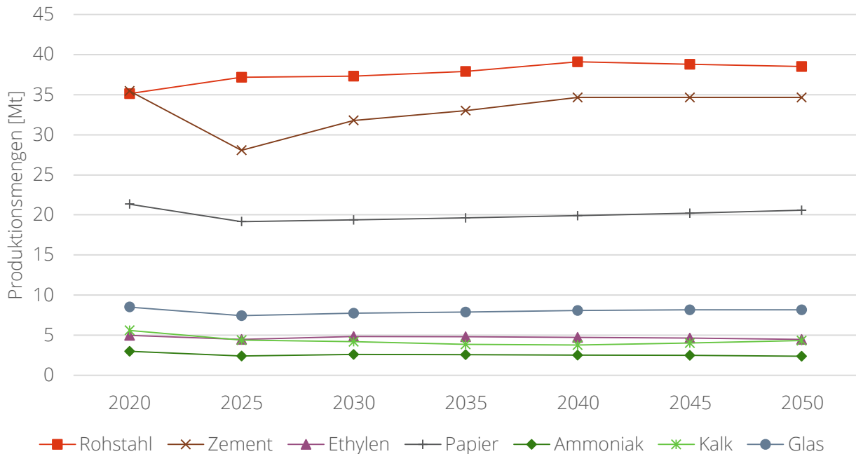
Abbildung A 22: Produktionsmengen für die energieintensiven Produkte Rohstahl, Zement, Ethylen, Papier, Ammoniak, Kalk und Glas
