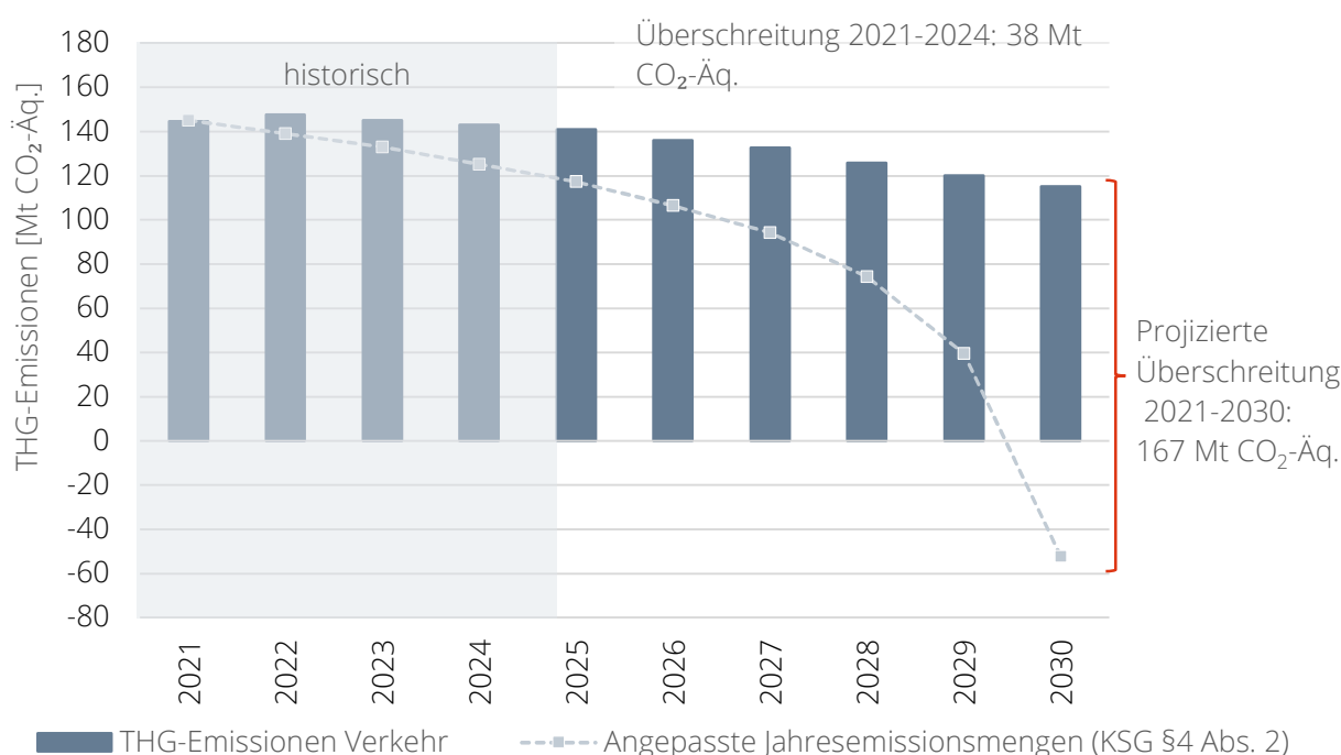
Abbildung 31: Entwicklung der historischen und projizierten THG-Emissionen im Sektor Verkehr
