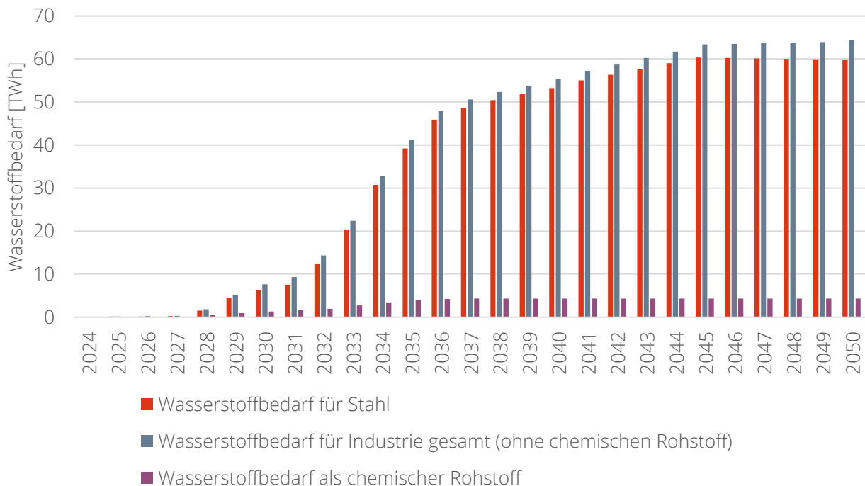
Abbildung A 23: Hochlauf Wasserstoffbedarf in der Industrie
