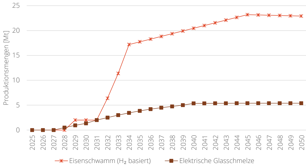
Abbildung A 26: Produktionsmengen CO 2 -arme/-freie Technologien Eisenschwamm und elektrische Glasschmelze
