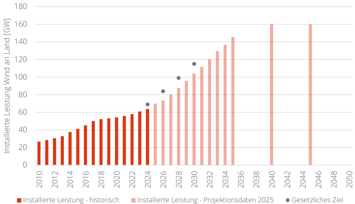
Abbildung A 13: Historische und projizierte Entwicklung der installierten Leistung von Wind an Land und die gesetzliche Zielsetzung
