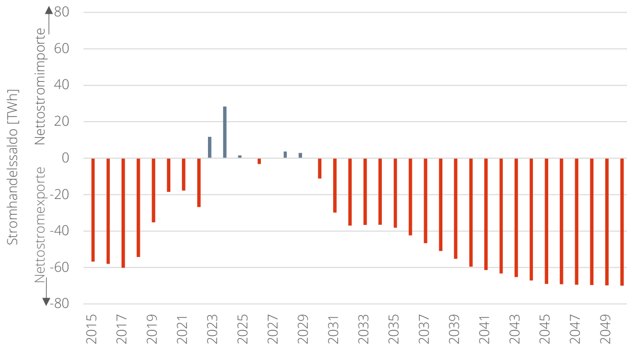
Abbildung A 9: Historische und projizierte Entwicklung des Stromhandelssaldos im Zeitverlauf
