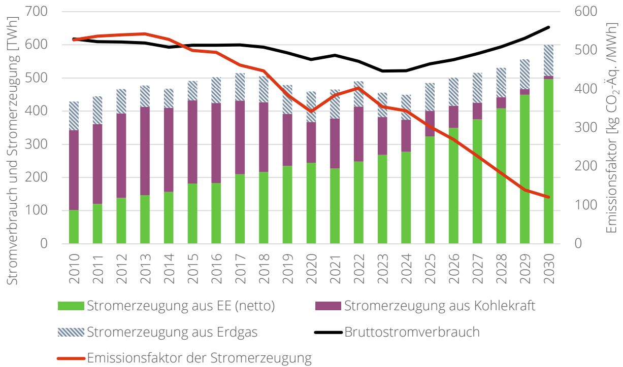
Abbildung A 7: Bruttostromverbrauch, Stromerzeugungsmix und Emissionsfaktor der Stromerzeugung im Zeitverlauf
