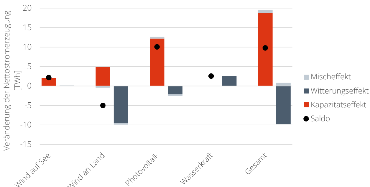
Abbildung A 16: Veränderung der Nettostromerzeugung aus erneuerbaren Energieträgern im Jahr 2024 gegenüber dem Vorjahr
