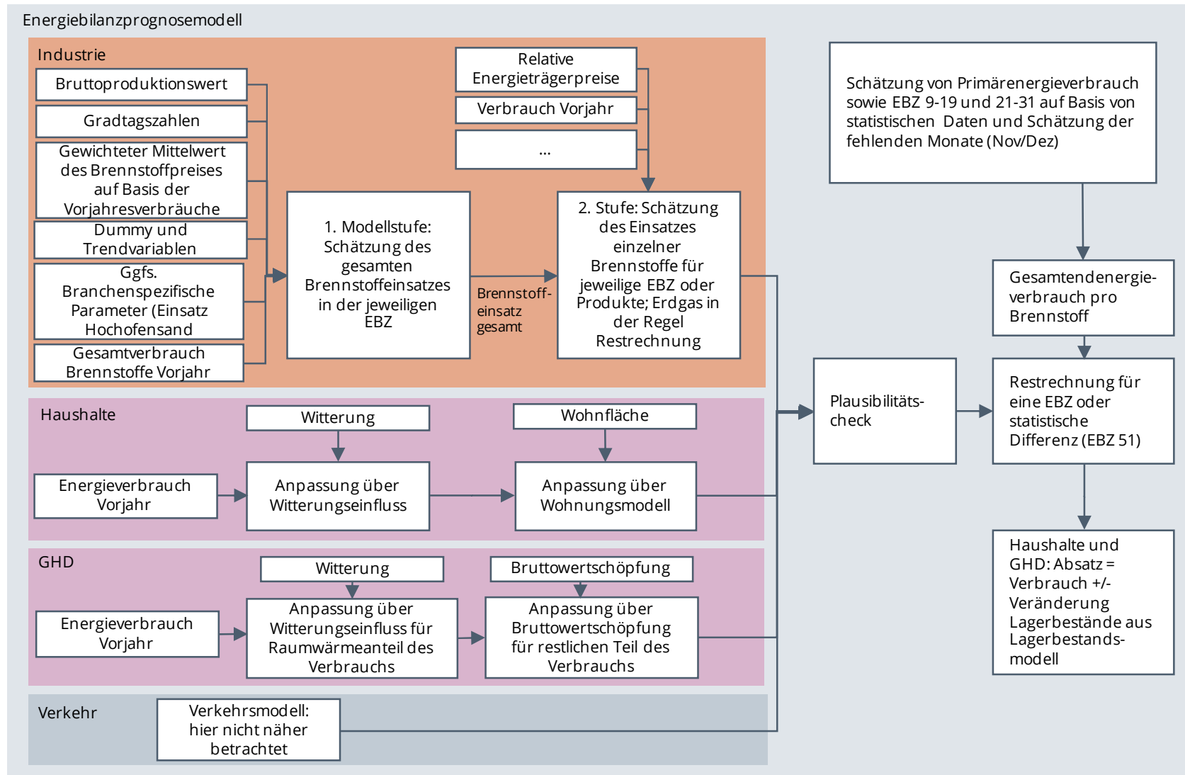
Abbildung 4: Schematische Darstellung des Energiebilanzprognosemodells der AGEB zur Berechnung der Frühschätzung der Energiebilanz
