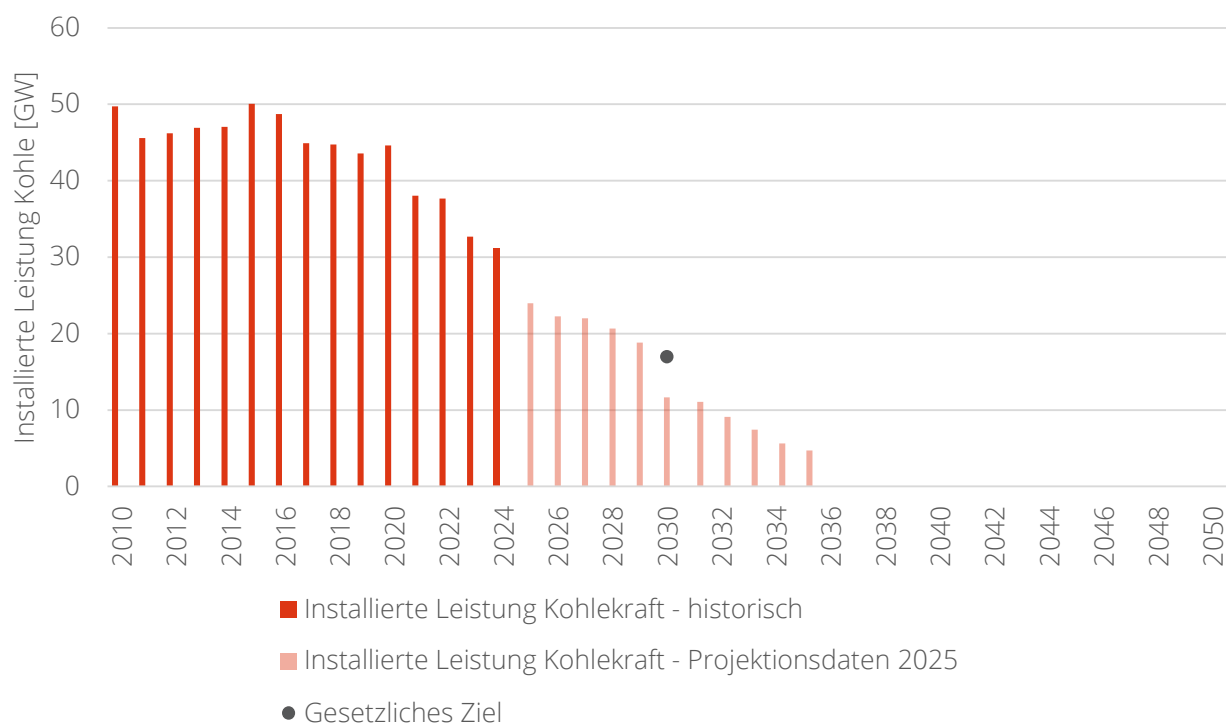
Abbildung A 10: Entwicklung der installierten Leistung von Braun- und Steinkohlekraftwerken, die gesetzliche Zielsetzung und die projizierte Entwicklung in den Projektionsdaten 2025
