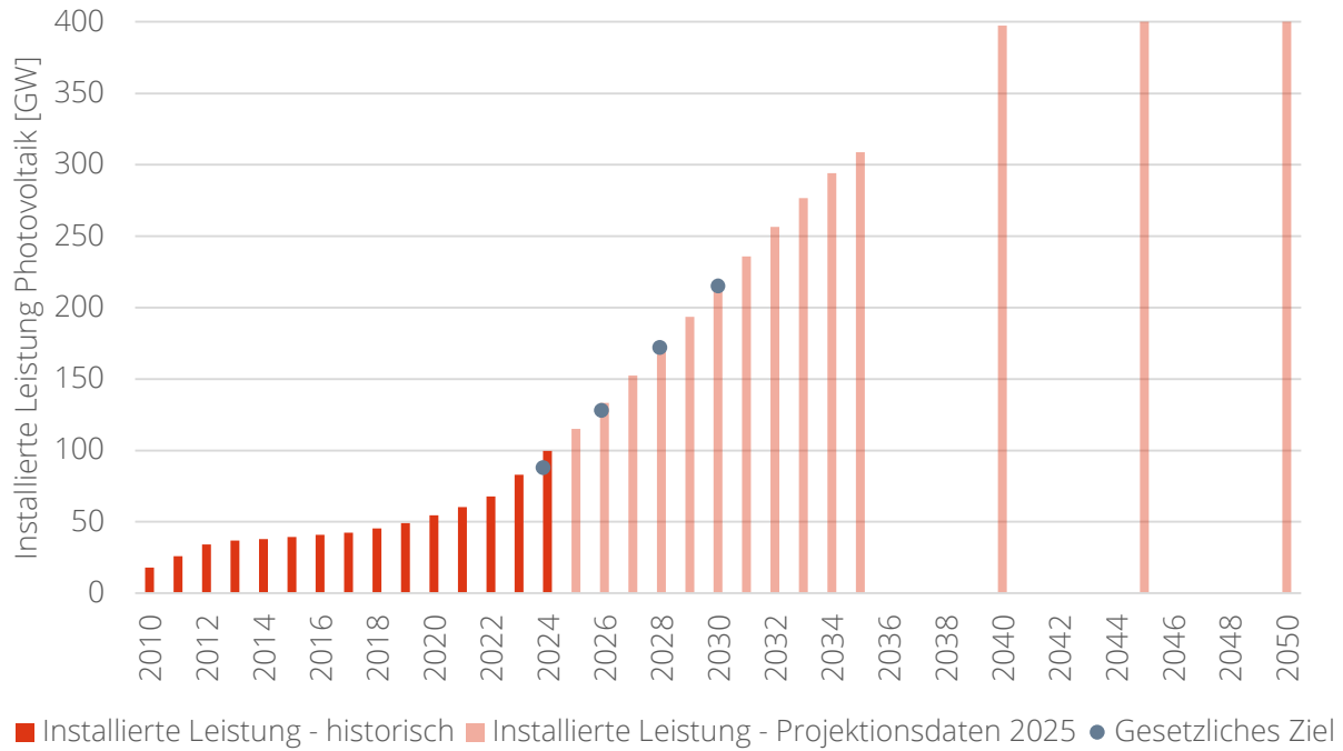
Abbildung A 15: Historische und projizierte Entwicklung der installierten Leistung der Photovoltaik und die gesetzliche Zielsetzung
