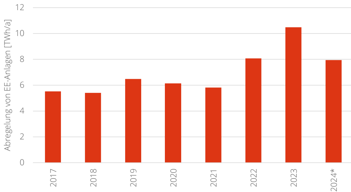
Abbildung A 17: Historische Abregelung von erneuerbaren Energieträgern von 2017 bis 2024
