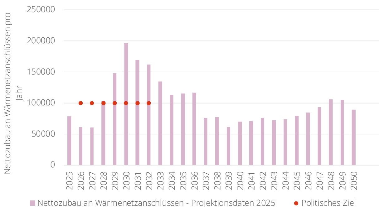
Abbildung 30: Historische und projizierte Entwicklung des Nettozubaus von Wärmenetzanschlüssen
