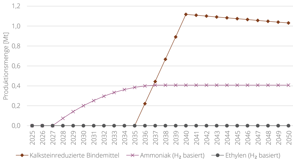
Abbildung A 25: Produktionsmengen CO 2 -arme/-freie Technologien Ammoniak, Ethylen und Kalksteinreduzierte Bindemittel
