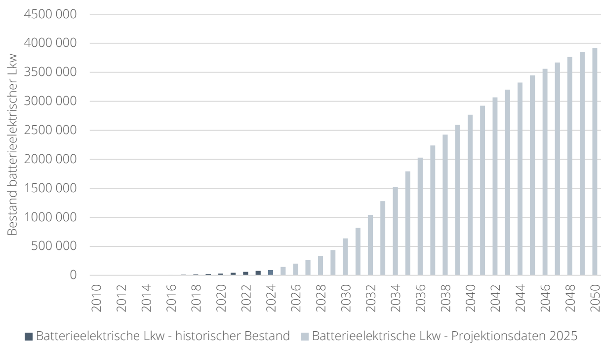
Abbildung A 34: Historischer Bestand batterieelektrischer Lkw und die projizierte Entwicklung in den Projektionsdaten 2025
