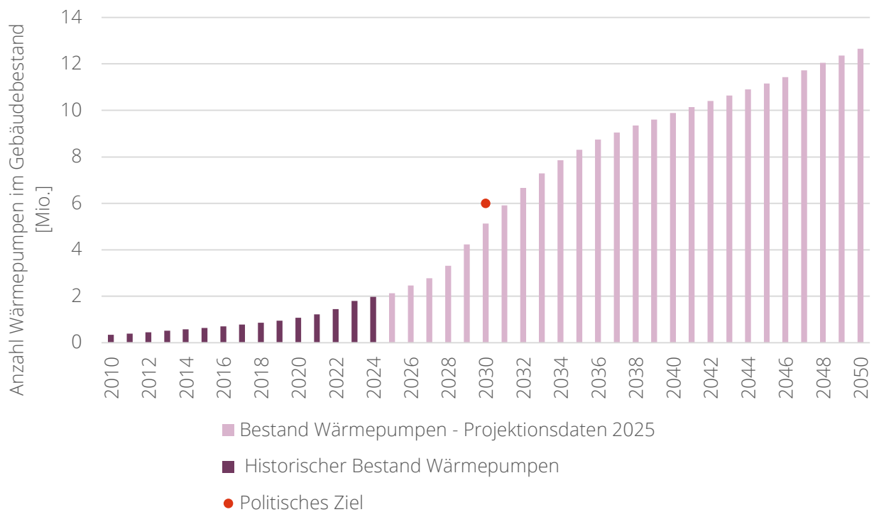
Abbildung A 30: Historische und projizierte Entwicklung des Wärmepumpenbestands in Gebäuden
