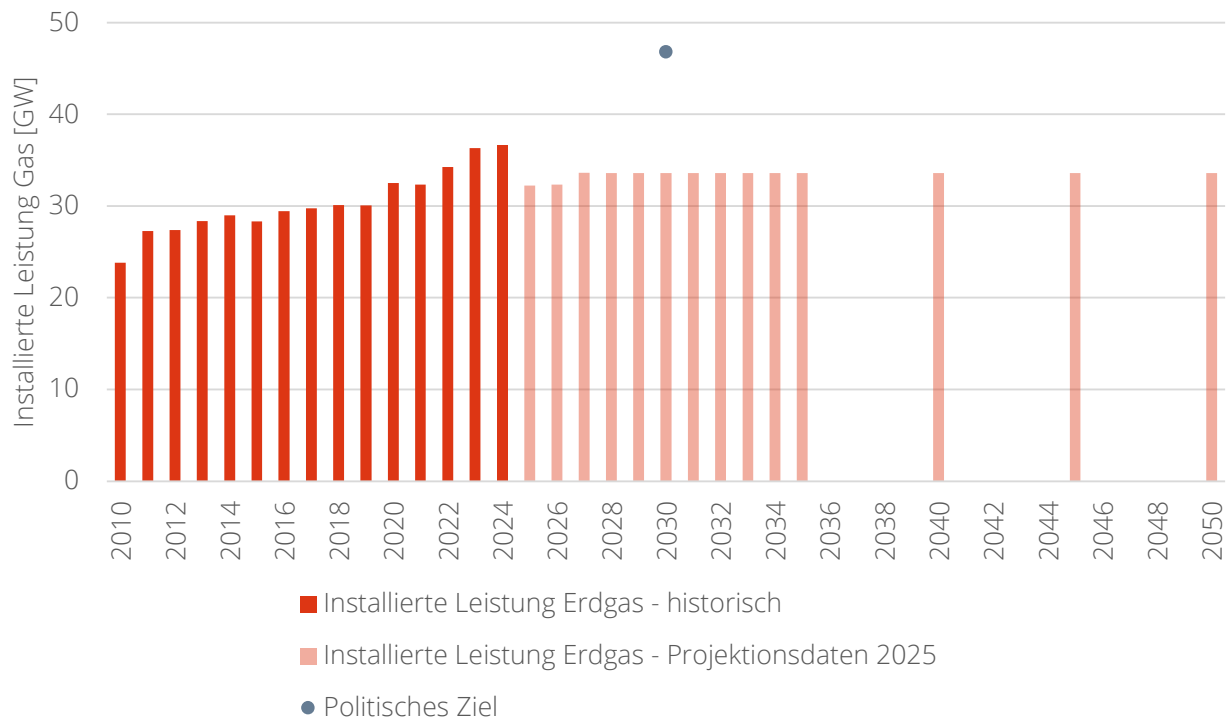
Abbildung A 11: Entwicklung der installierten Leistung von Erdgaskraftwerken, die politische Zielsetzung und die projizierte Entwicklung in den Projektionsdaten 2025
