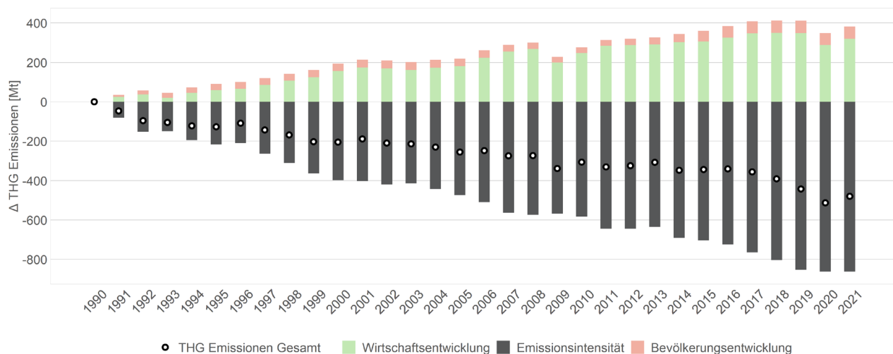
Abbildung 8: Dekomposition der Treibhausgasemissionen gesamt - Änderungen im Vergleich zu 1990
