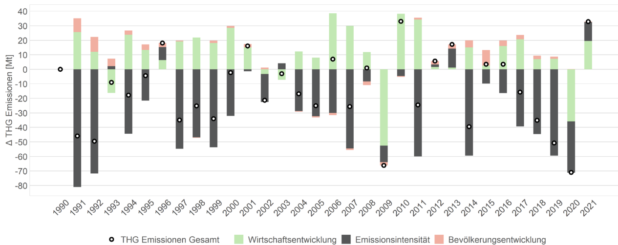
Abbildung Z-2: Dekomposition der Treibhausgasemissionen gesamt – Änderungen im Vergleich zum Vorjahr
